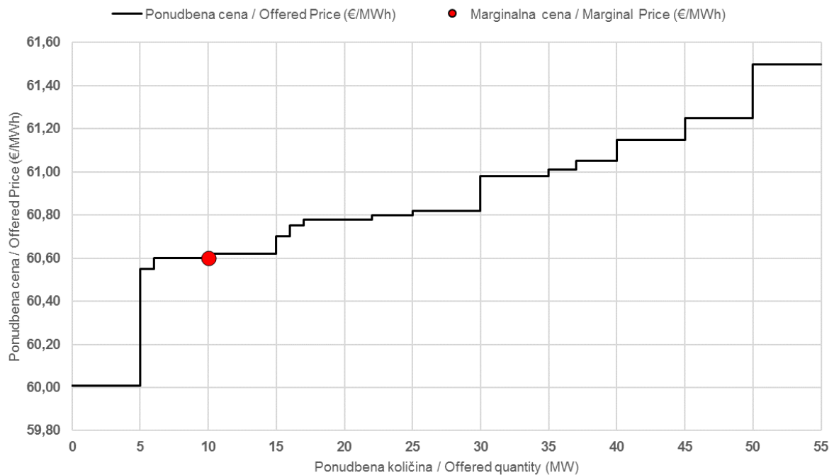
Slika 1: Agregatna krivulja ponudb za produkt pasovne energije za leto dobave 2020
