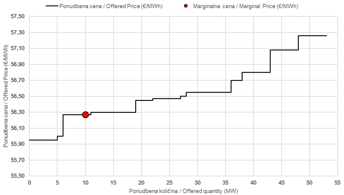
Slika 3: Agregatna krivulja ponudb za produkt pasovne energije za leto dobave 2022
