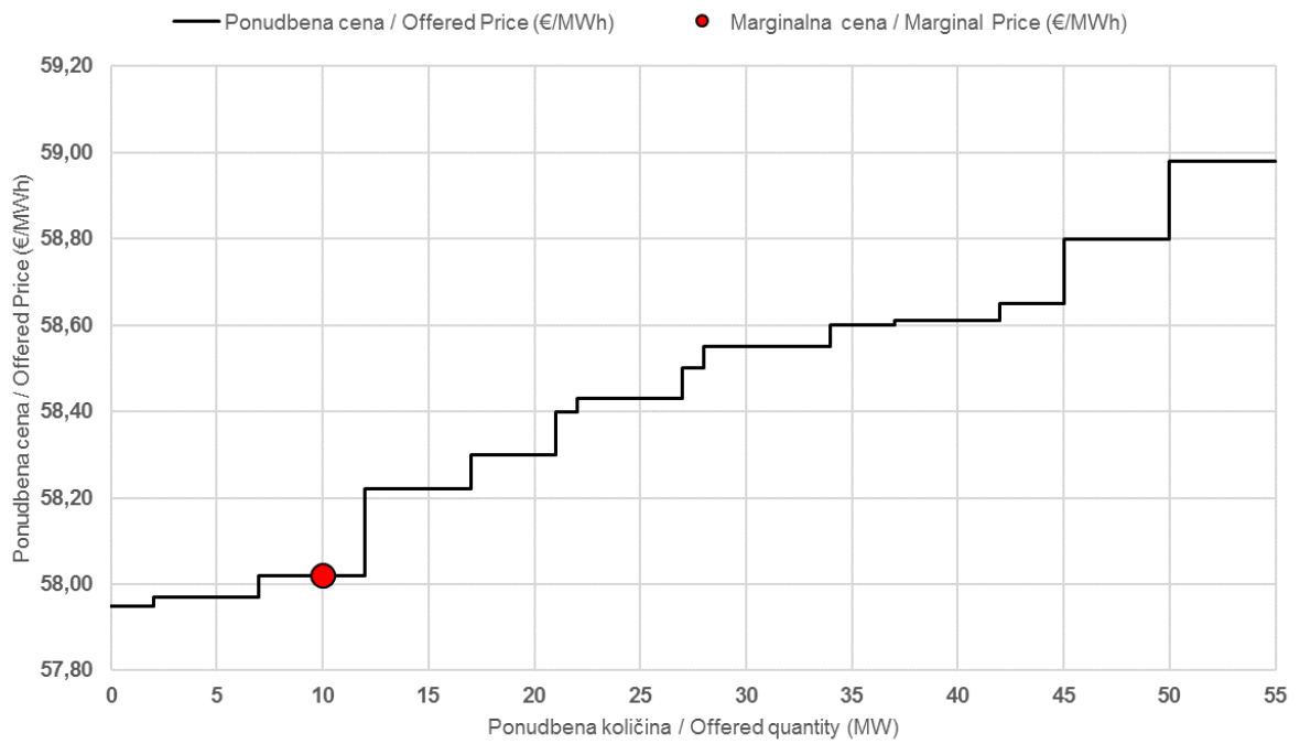
Slika 2: Agregatna krivulja ponudb za produkt pasovne energije za leto dobave 2021
